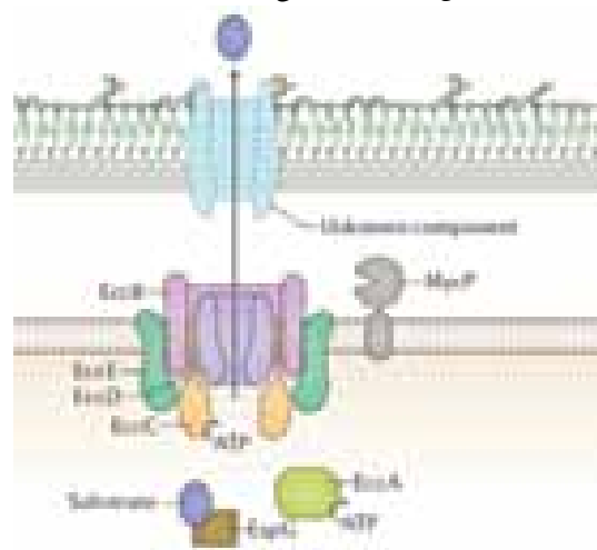
شکل ۲: نمایی از سیستم ترشحي تیپ VII در مایکوباکتریوم توبرکلوزیس
