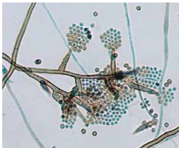
فیالوفورا ریچاردزیه
