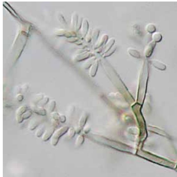
رینوکلادیدا آتروویرنس
