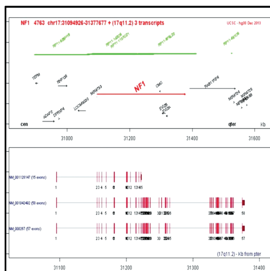
شکل ۹: بررسی NF در آزمایش WES
