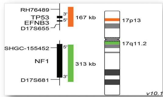
شکل ۲: مکان ژن مربوط به بیماری NF1 روی کروموزوم ۱۷ Metasystems-probes.com
